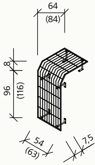
Rankgitter Typ A (Rückwand und Dach) für Einzelschrank 120S (240)
