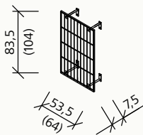
Rückwand
