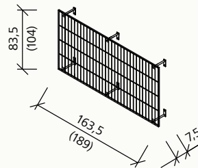
Rückwand
