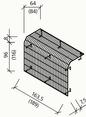
Rankgitter Typ A (Rückwand und Dach) für Dreifachschrank 120S (240)
