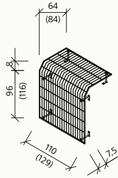
Rankgitter Typ A (Rückwand und Dach) für Doppelschrank 120S (240)
