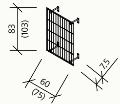
Rankgitter Typ B (Seitenwand) für Einzel-, Doppel- und Dreifachschrank 120 (240)
