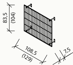
Rückwand
